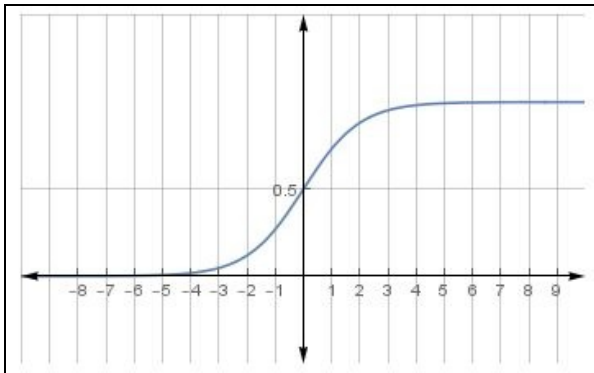
Sigmoid
