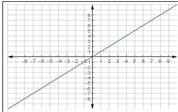
Linear
